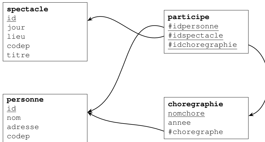
FIGURE 1 – Schéma relationnel de la base
