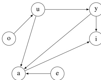
FIGURE 1 – Graphe de l'exemple
