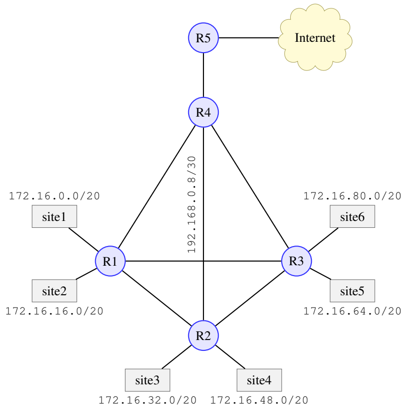
FIGURE 1 – Schéma du réseau du lycée
