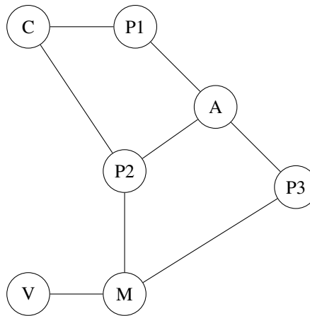
FIGURE 2 – Graphe des domiciles et points de rendez-vous
