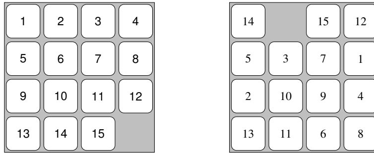
FIGURE 1 – Une grille rangée, à gauche, et mélangée, à droite
